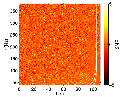
(d) EBBH B waveform
