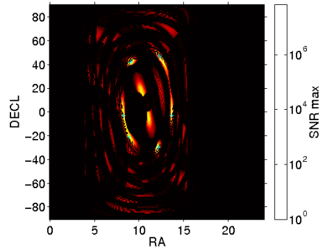
(d) Product of the above sky maps.
