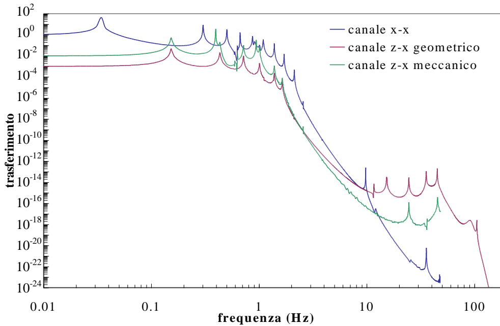
Figura 51 Canali di trasmissione effettiva della vibrazione orizzontale dal suolo allo specchio
