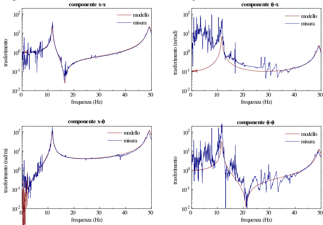
Figura 40 matrice di trasferimento 'orizzontale-angolare' dal vessel alla crossbar del filtro 0
