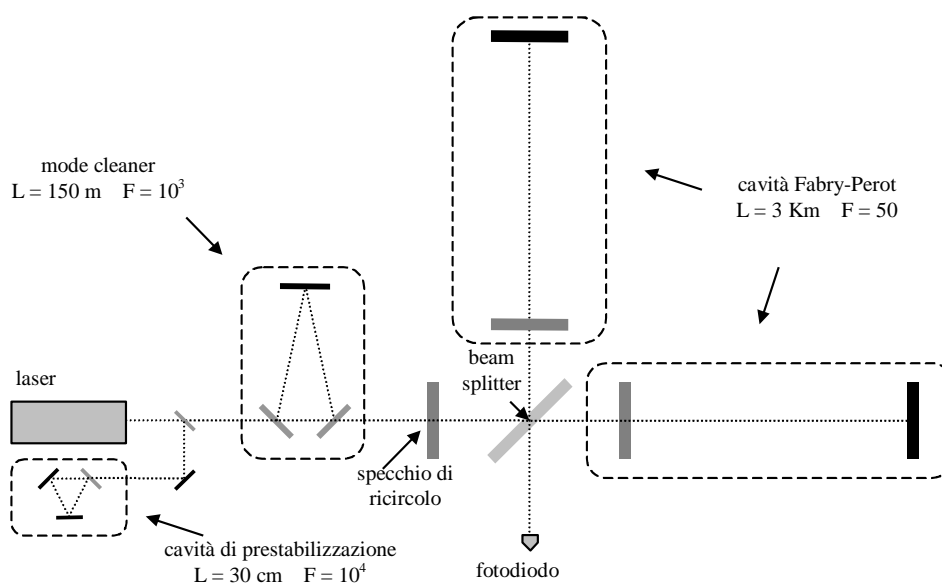
Figura 2 Rappresentazione schematica dell'interferometro VIRGO
