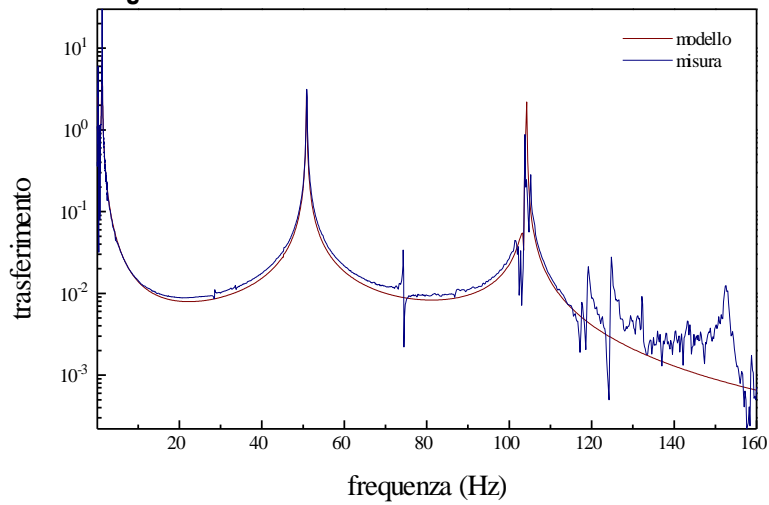
Figura 15 Funzione di trasferimento verticale del filtro 3
