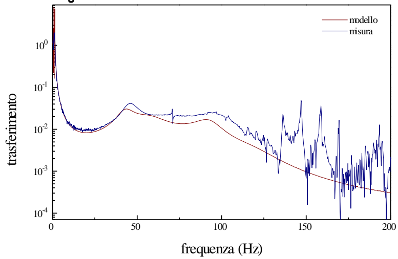
Figura 21 Funzione di trasferimento verticale del filtro 3
