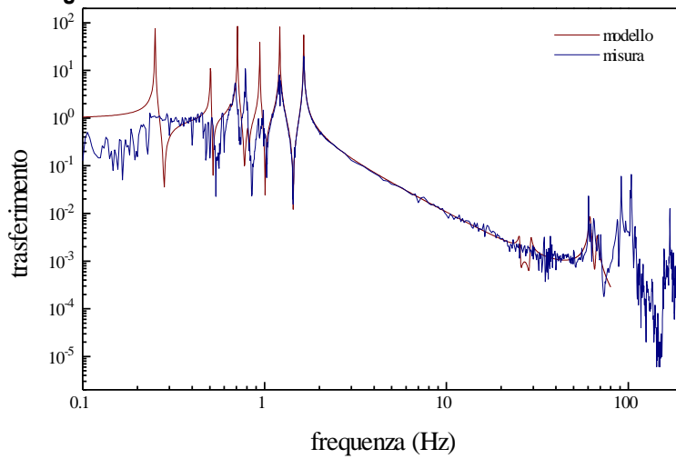
Figura 36 Funzione di trasferimento orizzontale del filtro 2
