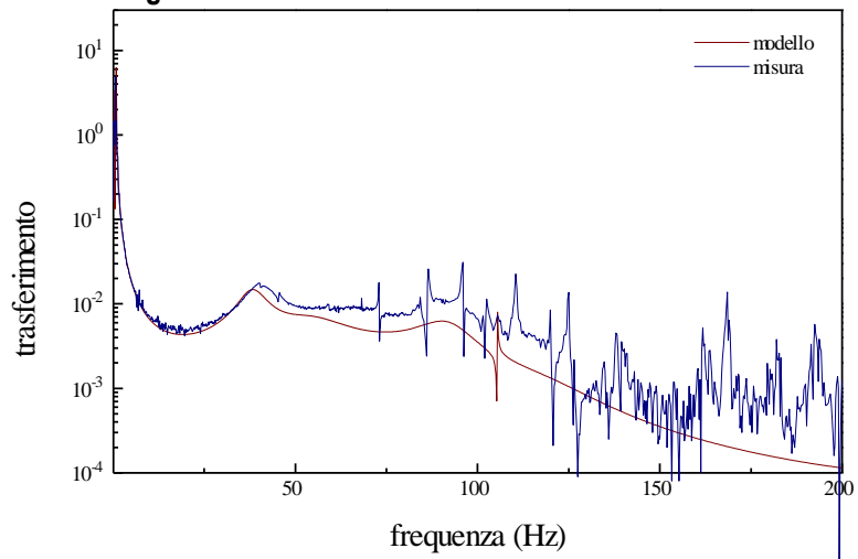
Figura 22 Funzione di trasferimento verticale del filtro 4
