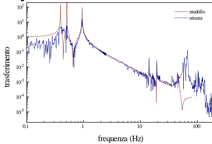
Figura 39 Funzione di trasferimento orizzontale del filtro 7
