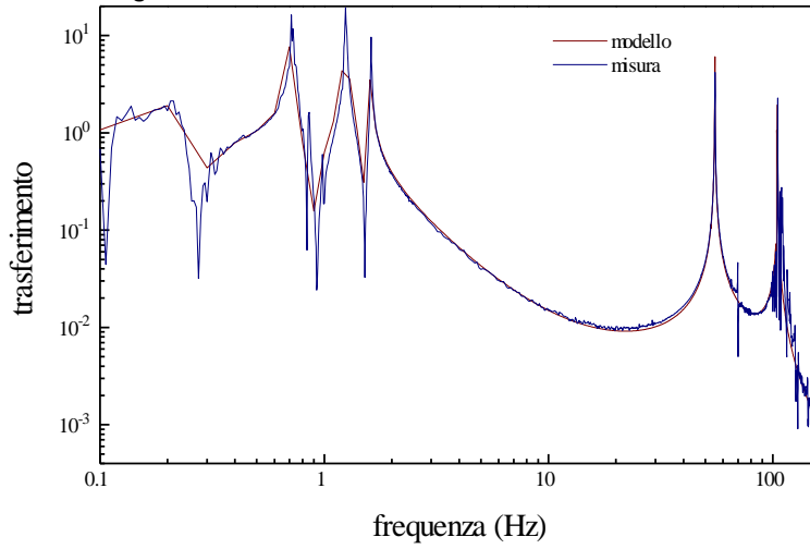
Figura 13 Funzione di trasferimento verticale del filtro 1
