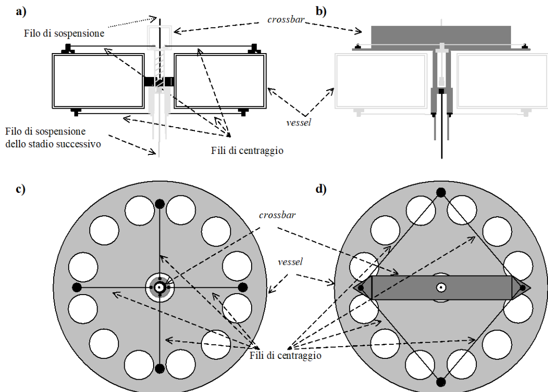
Figura 6 Filtro standard - a), b): sezioni laterali; c): vista inferiore; d): vista superiore
