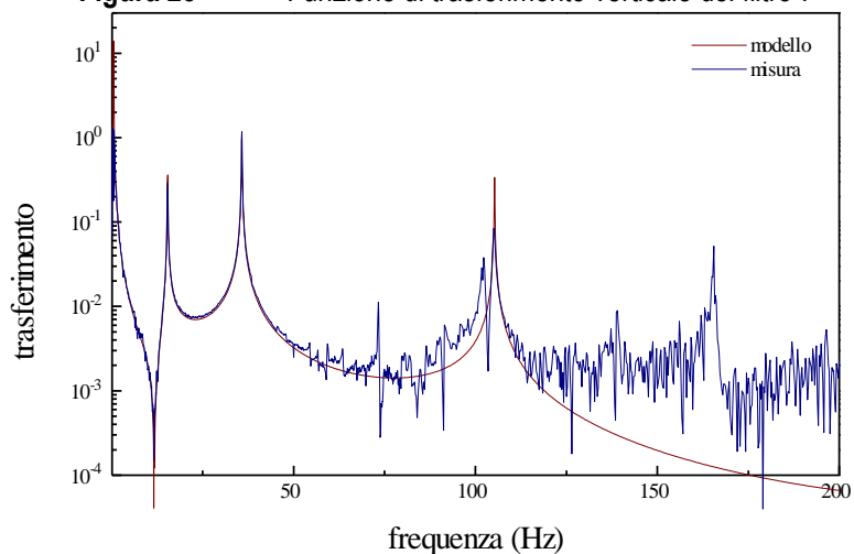
Figura 25 Funzione di trasferimento verticale del filtro 7
