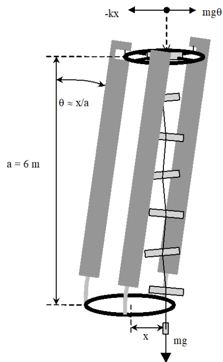
Figura 10 Rappresentazione schematica del pendolo invertito
