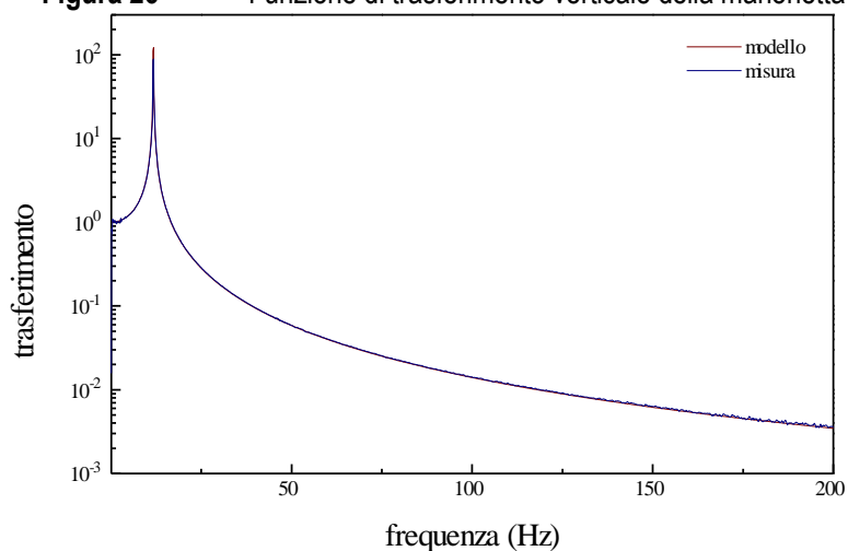
Figura 26 Funzione di trasferimento verticale della marionetta
