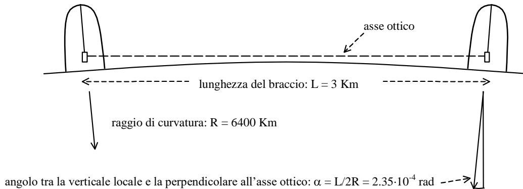
Figura 5 Incidenza della curvatura terrestre sulla trasmissione del rumore sismico
