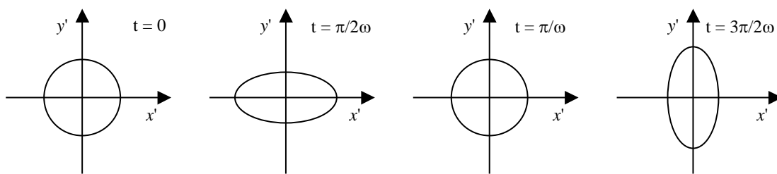
Figura 1 Moto di un anello di masse libere nel campo di un'onda gravitazionale polarizzata \epsilon_+^{TT}
