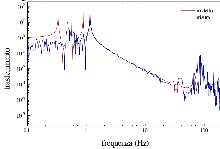
Figura 38 Funzione di trasferimento orizzontale del filtro 4
