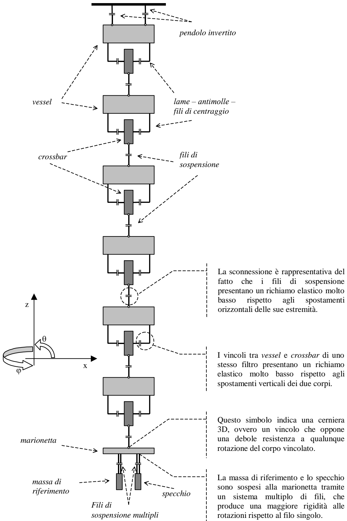
Figura 12 Rappresentazione schematica del superattenuatore
