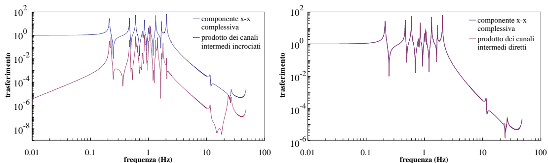
Figura 45 trasferimento orizzontale del filtro 0 e del filtro 1 combinati
