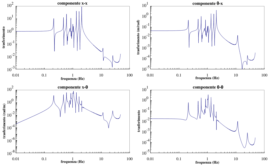
Figura 43 matrice di trasferimento 'orizzontale-angolare' del filtro 0
