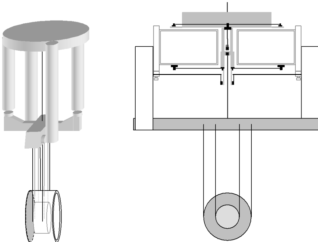
Figura 9 Stadio finale della sospensione (filtro 7 – marionetta – specchio)
