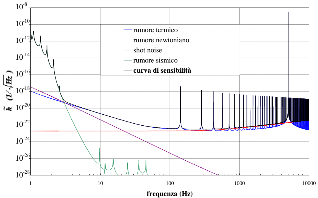
Figura 3 Densità spettrale lineare, in termini del campo equivalente, dei principali rumori in VIRGO
