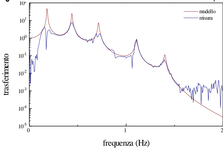
Figura 27 Funzione di trasferimento verticale dal filtro 1 allo specchio
