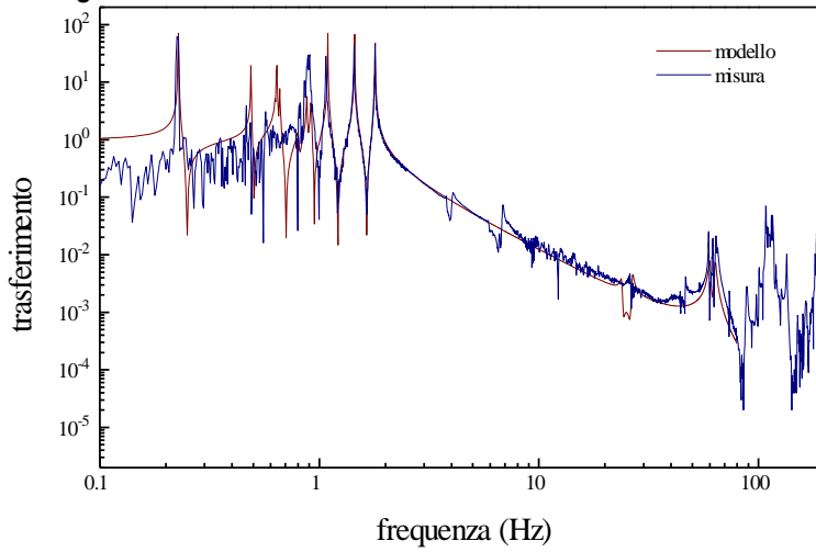
Figura 35 Funzione di trasferimento orizzontale del filtro 1
