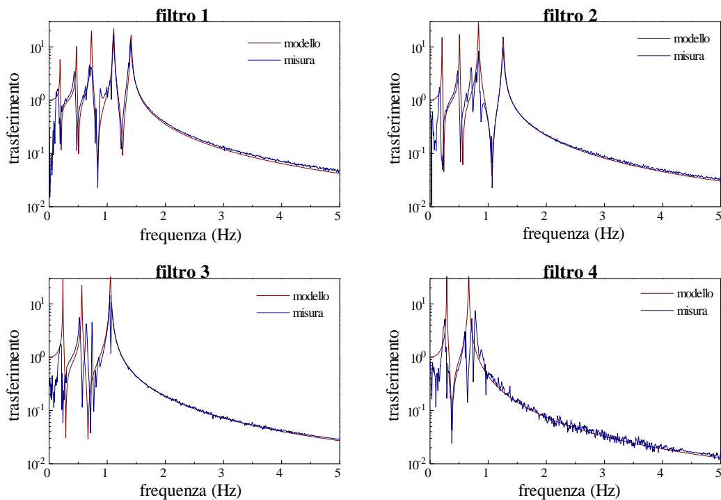
Figura 28 Funzione di trasferimento verticale in bassa frequenza dei filtri standard
