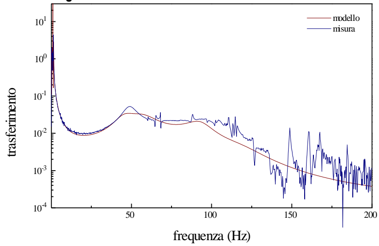
Figura 20 Funzione di trasferimento verticale del filtro 2
