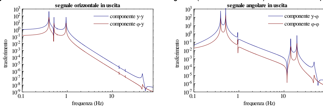
Figura 48 Matrice di trasferimento orizzontale-angolare (direzione trasversa) dal filtro 7 allo specchio
