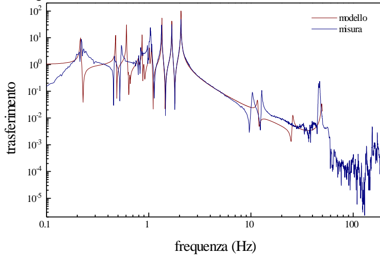
Figura 34 Funzione di trasferimento orizzontale del filtro 0
