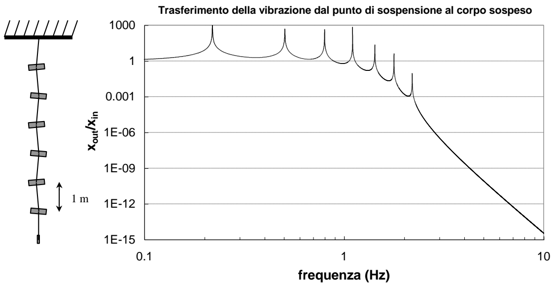
Figura 4 Pendolo multiplo come sistema di attenuazione delle vibrazioni
