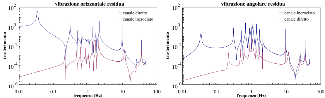
Figura 44 Trasferimento effettivo dal filtro 0 al filtro 1
