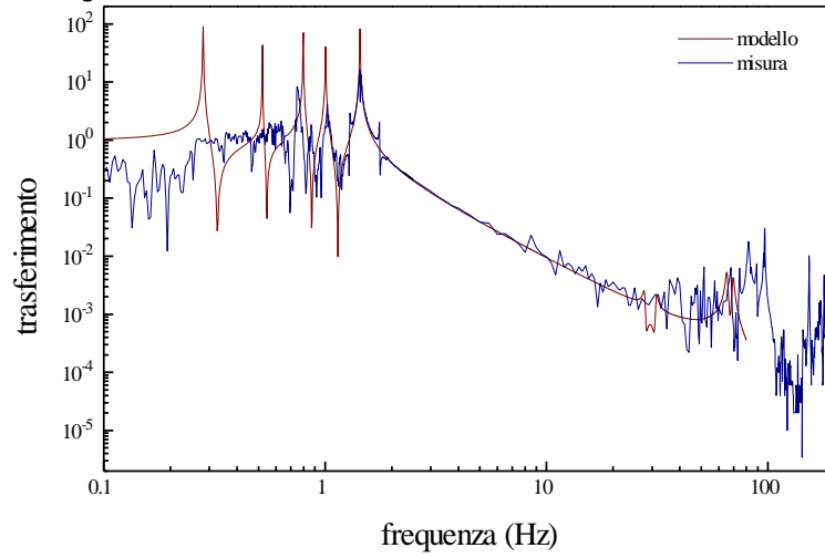
Figura 37 Funzione di trasferimento orizzontale del filtro 3
