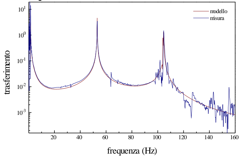
Figura 14 Funzione di trasferimento verticale del filtro 2
