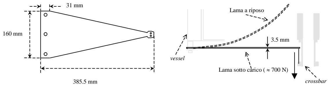
Figura 7 Lama triangolare precurvata
