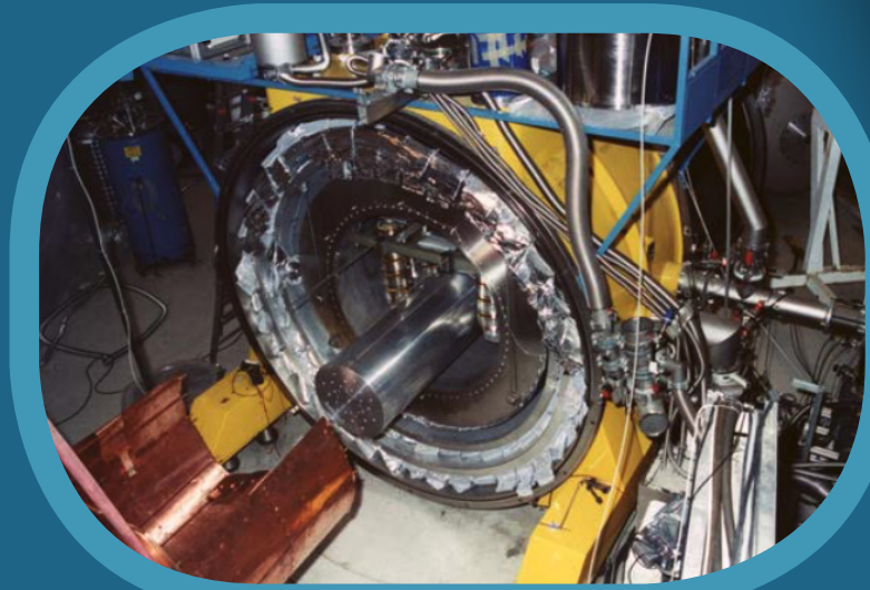
AURIGA nei Laboratori Nazionali di Legnaro
